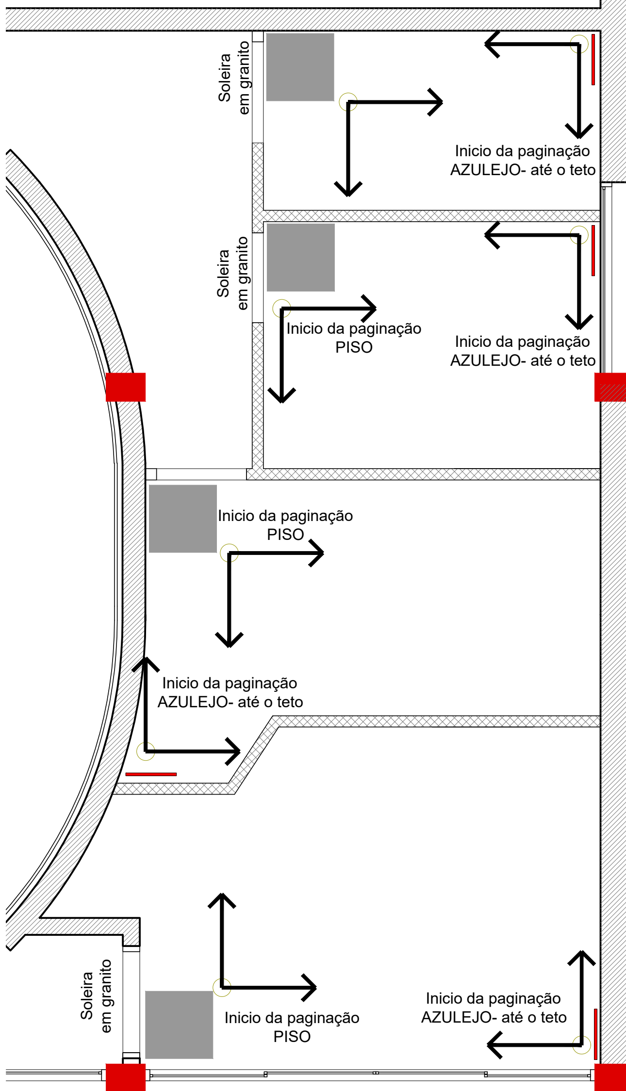
PLANTA BAIXA- SANITÁRIO E COPA ESC.: 1/75
