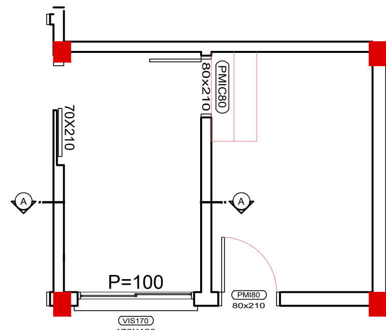
PLANTA BAIXA Esc.: Sem esc.
